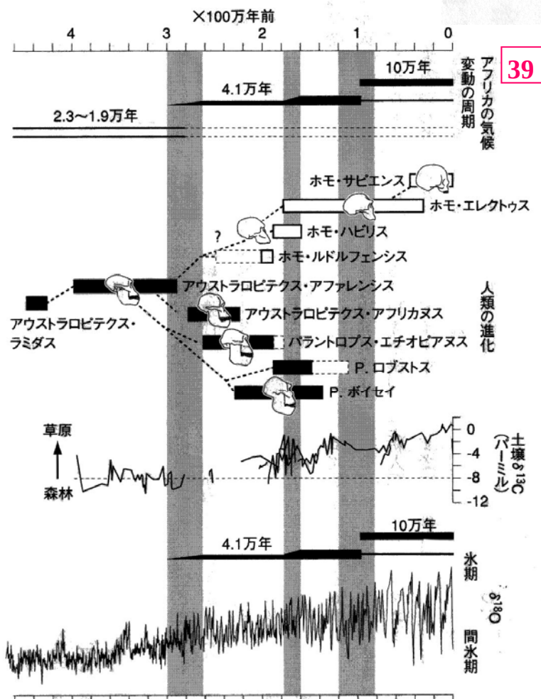
図52 人類進化と地球環境の変動 アフリカの気候変動の卓越周期の変遷、人類の進化、古土壌中の炭酸塩鉱物の炭素同位体比、海水酸素同位体比の変動と卓越周期の変化。deMenocal (1995) Science, 270, 53-59より。
